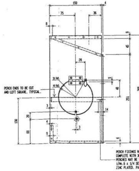
END ELEVATION
